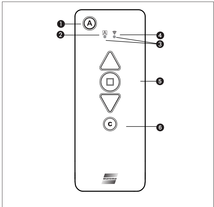
Abb. 13 Bedienfeld des WMS Handsenders basic
