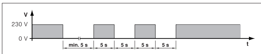
Abb. 25 PowerUp am WMS Zwischenstecker
