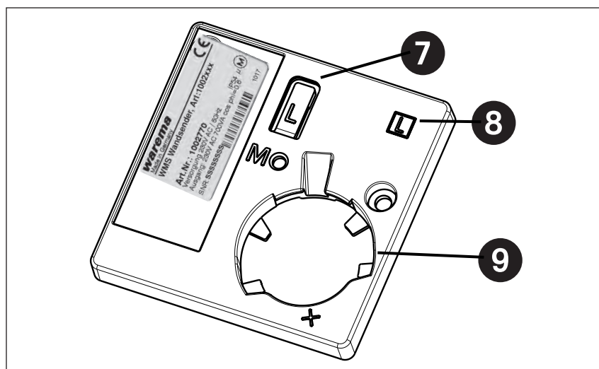
Abb. 16 Rückseite des WMS Wandsender
