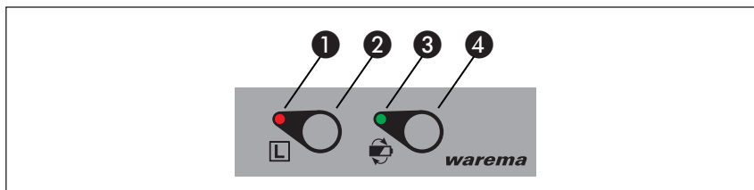
Abb. 21 Bedienfeld des WMS Windsensors
